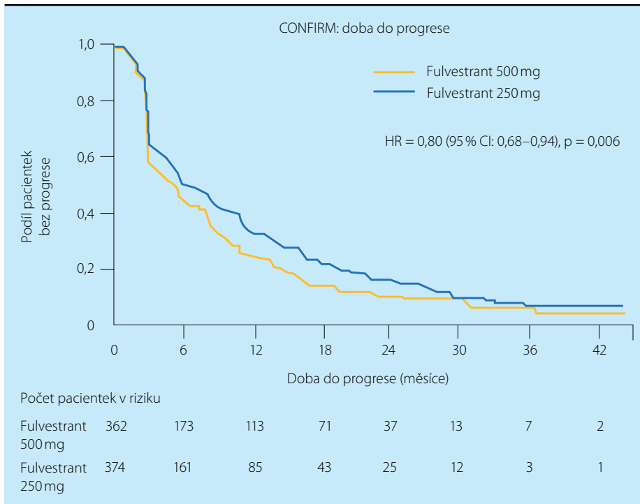
Graf 3. Doba do progresie onemocnení studie CONFIRM
